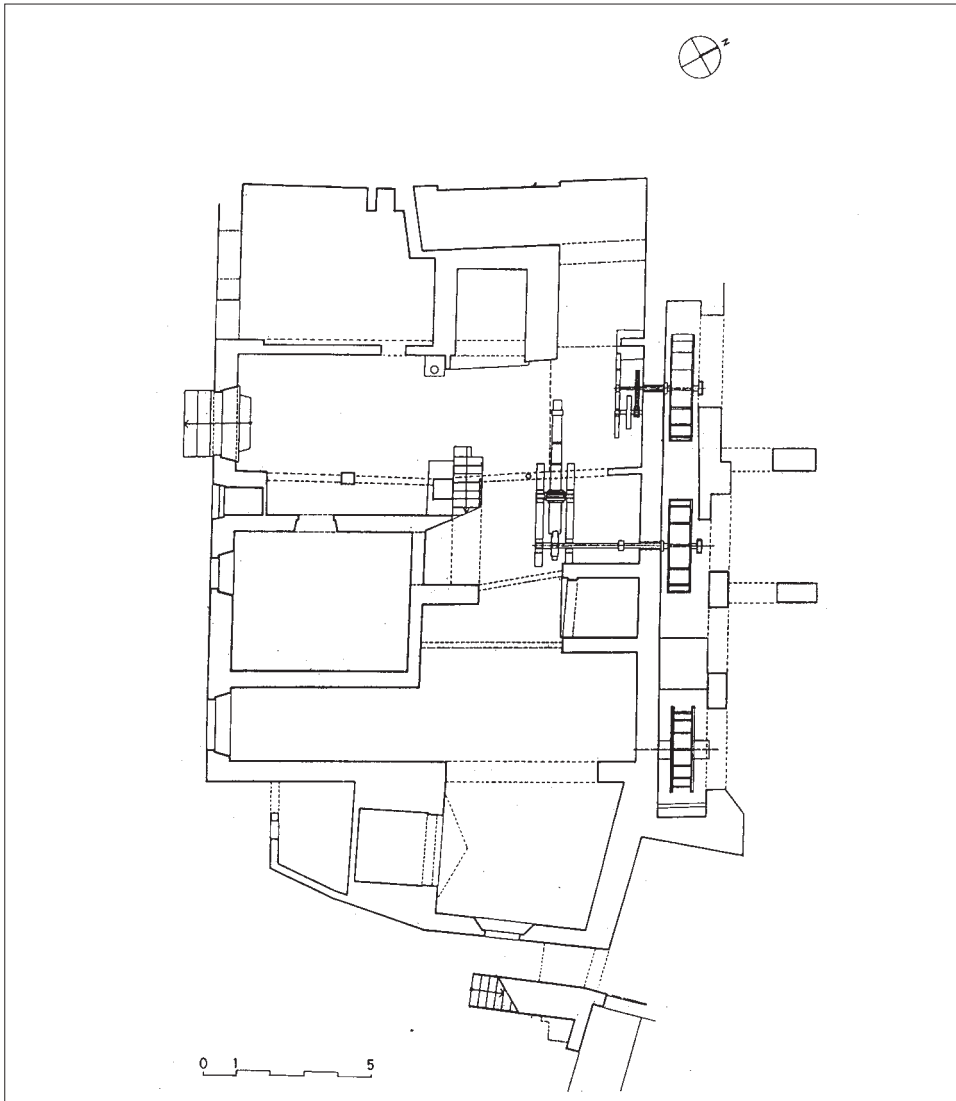
Dibuix de la farga de Banyoles, R. Lluch, J. Moner, Ll. Privat, "La farga de Banyoles...", pàg. 151. En la planta es mostra el funcionament de la maquinària.
